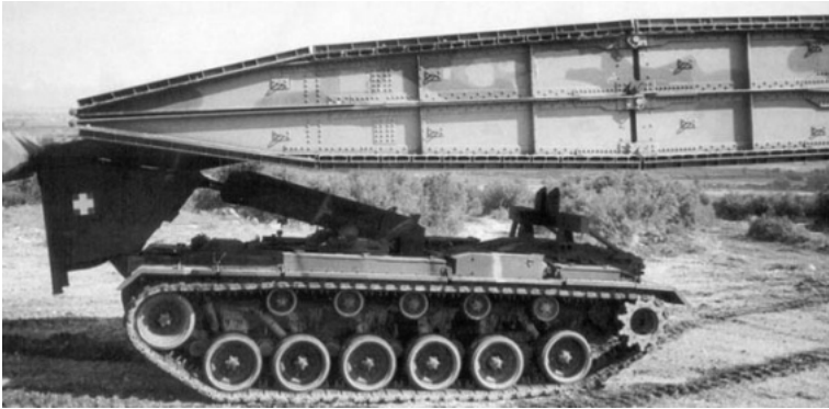
Véhicules poseurs de ponts M48 et M60.
